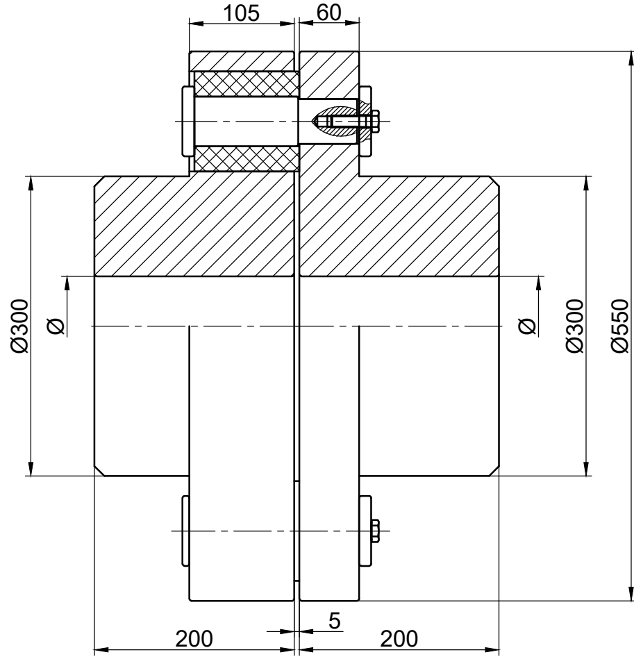
A-A KESİTİ
