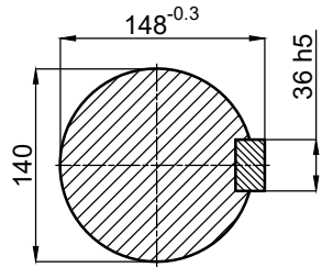
A-A KESİTİ
