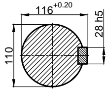
A-A KESİTİ
